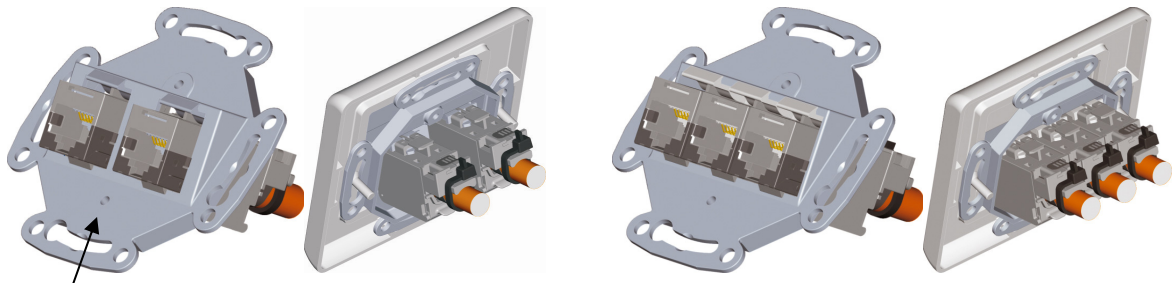
M4 Gewinde für PA - Anschluss
